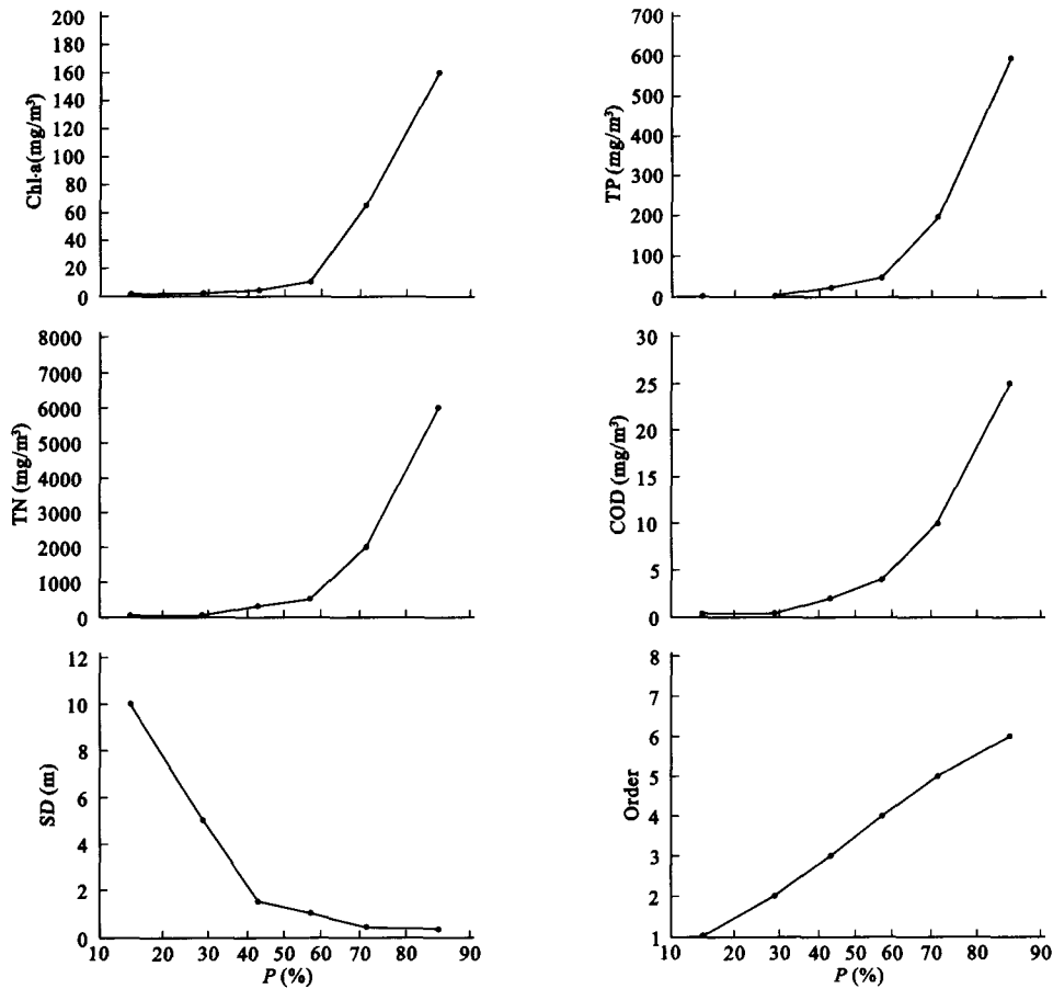
图 1 水质指标及评价级别的经验频率曲线
