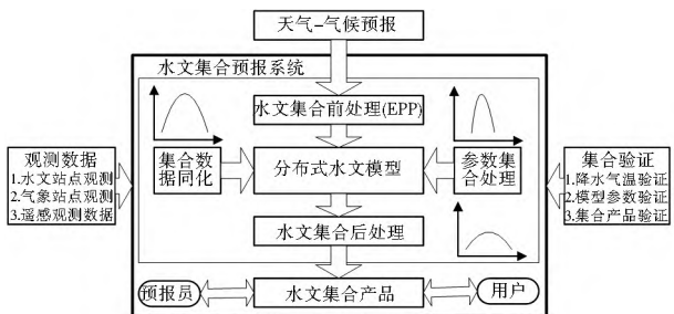
图 1 水文集合预报系统结构
